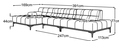
REC Armteil links + Element 105 (RVM) + 2HT rechts (RVM) Bestell-Nummer: D115631
