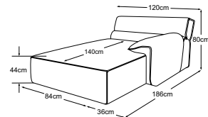
REC rechts Bestell-Nummer: D009122
