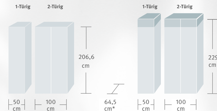
Korpus und Inneneinteilung
