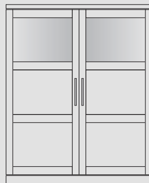
BI-023B Highboard 2-trg. Innen: 2 Holzfachböden, BE-161 Beleuchtungsset H/B/T: 150 x 120 x 41
