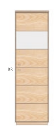
AX - 6102 R Vitrine 1+1-trg. rechts angeschlagen 4x HB, 1x KB, BE-001 H/B/T: 192x56x40
