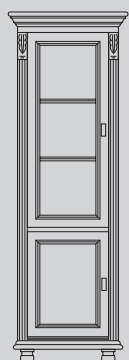
IND-008L Vitrine 1+1 trg. Türen links angeschlagen, Innen: oben 2 Holzfachböden, unten 1 Holzfachboden H/B/T: 192 x 62 x 45 AD-120 Beleuchtungsset für IND-008 IND-009L Schrank 1+1 trg. wie IND-008L jedoch obere Türe mit Holzfüllung H/B/T: 192 x 62 x 45
