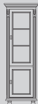
IND-008R Vitrine 1+1 trg. Türen rechts angeschlagen, Innen: oben 2 Holzfachböden, unten 1 Holzfachboden H/B/T: 192 x 62 x 45 AD-120 Beleuchtungsset für IND-008 IND-009R Schrank 1+1 trg. wie IND-008R jedoch obere Türe mit Holzfüllung H/B/T: 192 x 62 x 45
