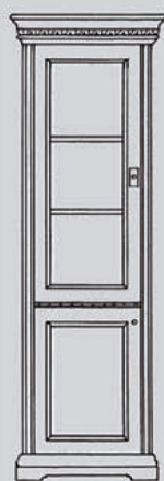
AD-008L Vitrine 1+1 trg. Türen links angeschlagen, Innen: oben 2 Holzfachböden, unten 1 Holzfachboden H/B/T: 190 x 64 x 44 AD-120 Beleuchtungsset für AD-008
