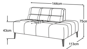
2HT rechts inkl. RVM Bestell-Nummer: D130521
