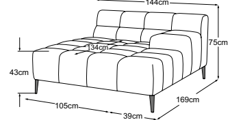
REC Armteil rechts Bestell-Nummer: D130131
